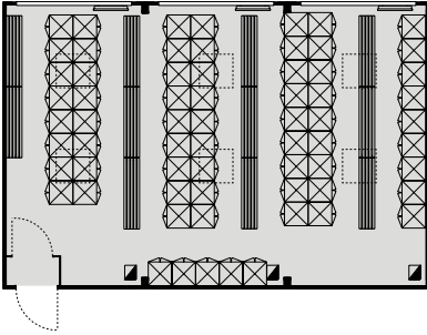
3 prémiové kontejnery (každý o šířce 3 metry) 66 osob
