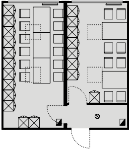
2 prémiové kontejnery (každý o šířce 3 metry) 12 osob 8 osob
