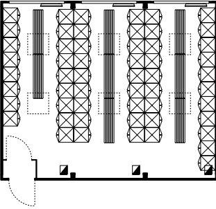
3 univerzální kontejnery (každý o šířce 2,5 metru) 55 osob
