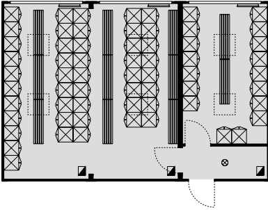
3 prémiové kontejnery (každý o šířce 3 metry) 45 osob 17 osob
